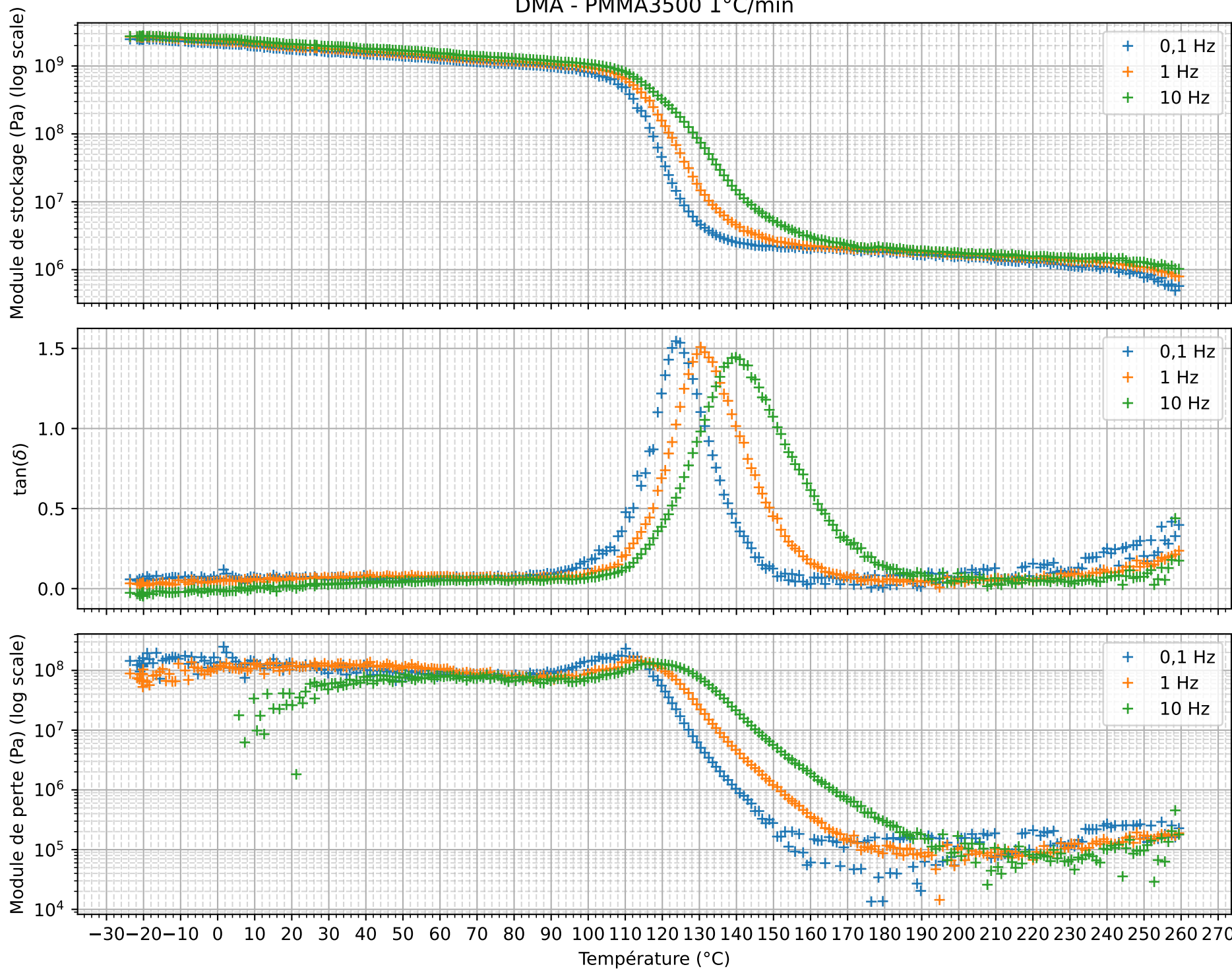
DMA - PMMA3500 1°C/min
